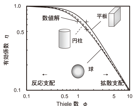
図7 各種形状におけるThiele数と触媒有効係数の関係(1次反応)(数値解は例題23, 24のもの)
