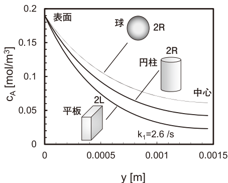
図4 球，円柱，平板状触媒の濃度分布比較
