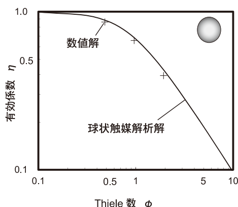
図6 Thiele数と触媒有効係数の関係(球状触媒, 1次反応)
