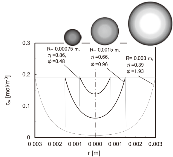
図5 球状触媒の濃度—形状の影響—
