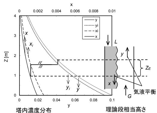
図10 吸収塔における理論段相当高さ
