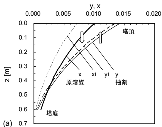
図6 塔型抽出プロセスの濃度分布, 操作線<cem04.xls>
