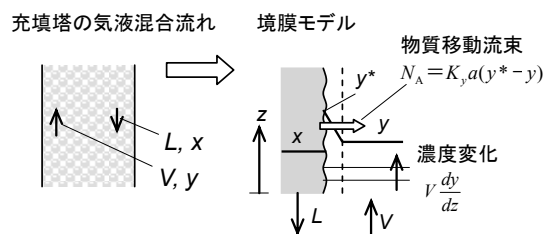
図8 充填塔蒸留の微分モデル
