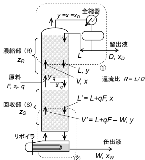
図7 充填塔による2成分系蒸留モデル
