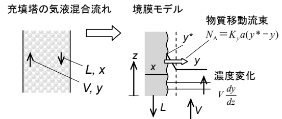
図8 充填塔蒸留の微分モデル
