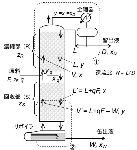
図7 充填塔による2成分系蒸留モデル
