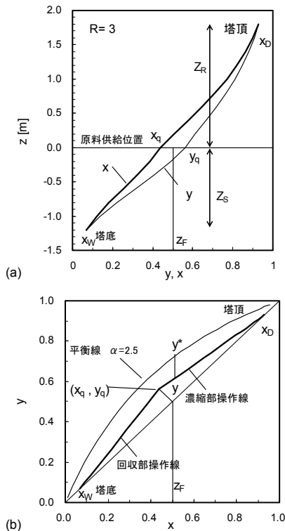
図9 充填塔による2成分系蒸留, (a) 塔内濃度分布と充填層高さ, (b) 操作線
